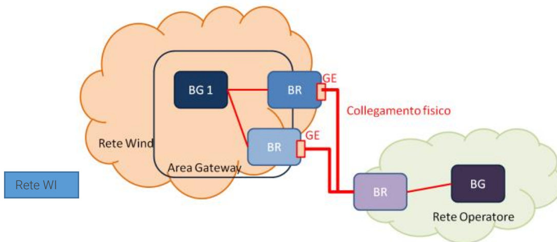
Figura 2: Modello architetturale d'interconnessione IP previsto da Welcome Italia
